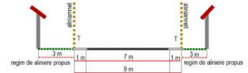
SECTIUNEA S7
