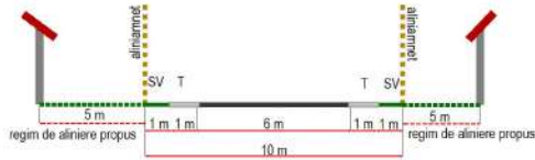
SECTIUNEA S4
