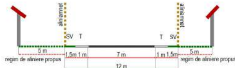
SECTIUNEA S8
