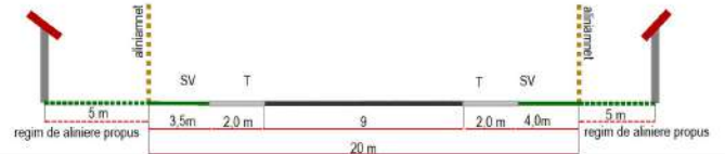
SECTIUNEA S13
