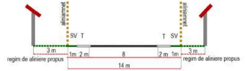
SECTIUNEA S12
