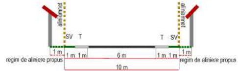
SECTIUNEA S6
