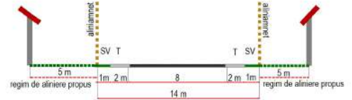
SECTIUNEA S11
