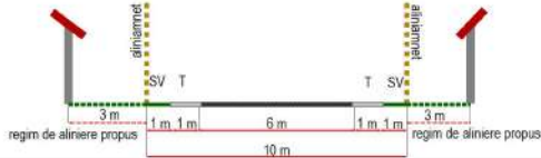
SECTIUNEA S5
