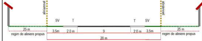
SECTIUNEA S14
