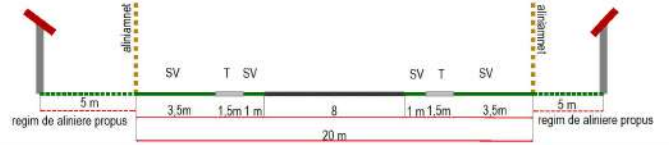
SECTIUNEA S10
